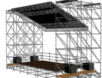
PALCO - VISTA PROSPETTICA
